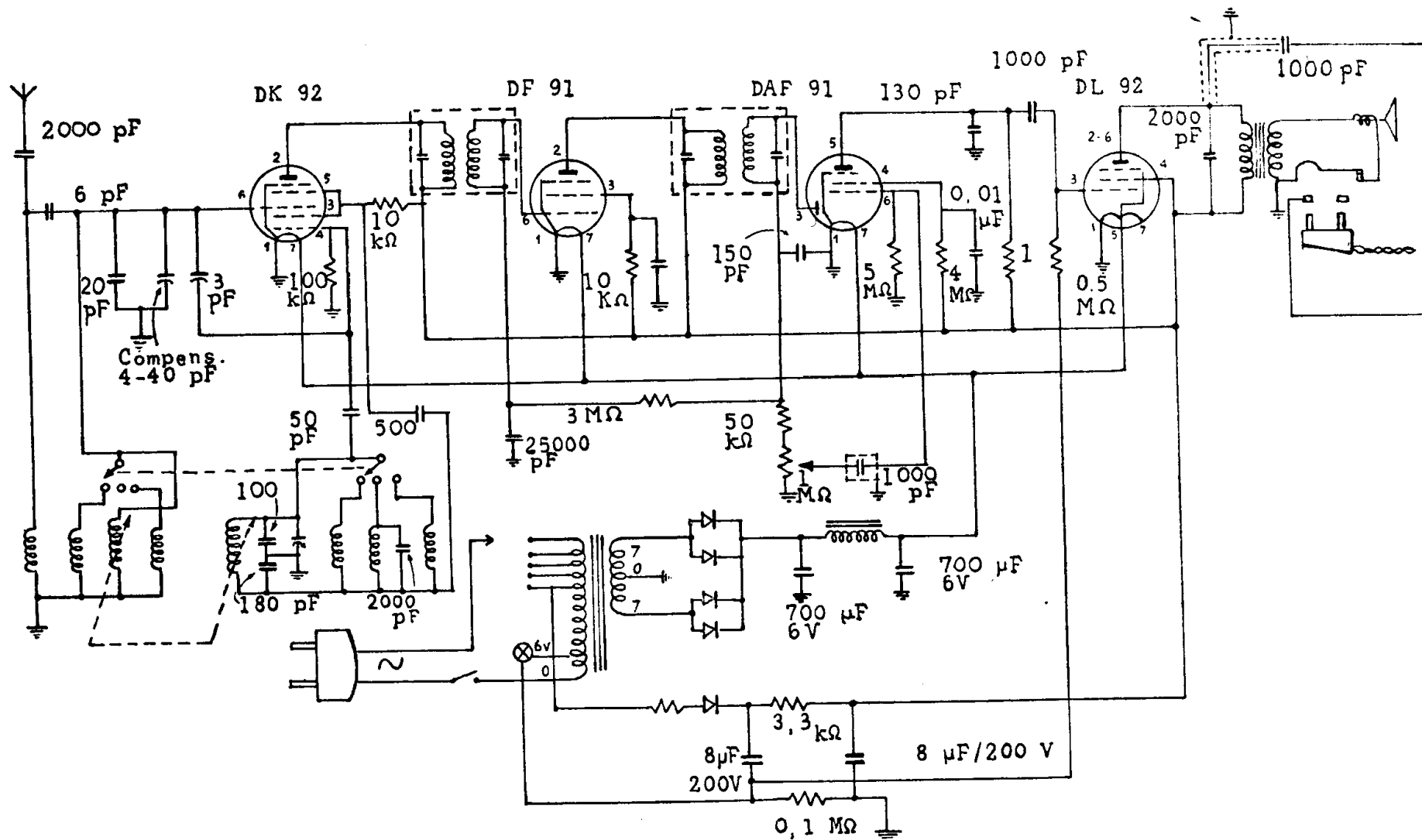
ALLOCCIO BACCHINI - Mod. Junior III per sola alimentazione in corrente alternata. Onde medie e due gamme onde corte. Media frequenza a 465 kc/s. Potenza d'uscita 200 milliwatt.
